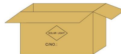
NUMĂRUL STRATULUI
