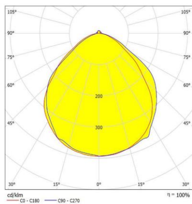
Distribuția Luminanței
